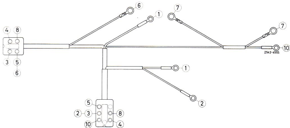
Bild 67-1/23 Zusatzleitungssatz (3) bei allen Typen außer den Limousinen der Typen 250 S bis 300 SEL/8 6.3
