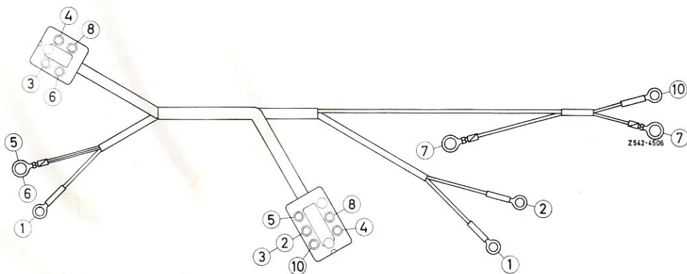
Bild 67-1/24 Zusatzleitungssatz (3) bei den Limousinen der Typen 250 S bis 300 SEL/8 6.3
